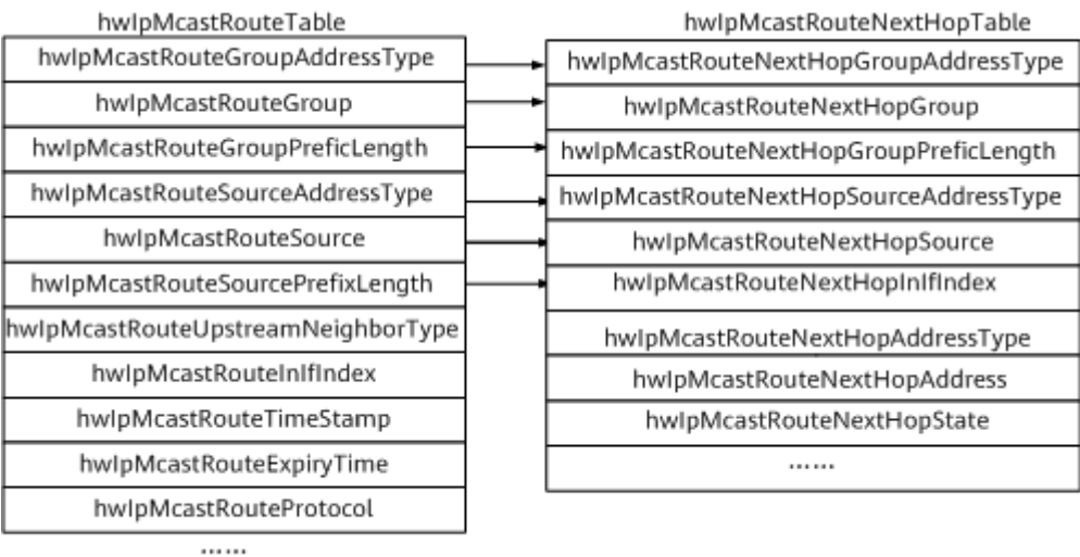
图 63-1 组播路由表和组播路由出接口表的表间关系图
